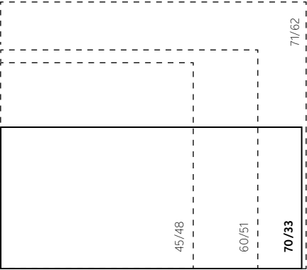
Dimensions de la vitre des foyers frontaux
