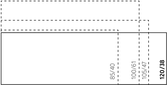
Dimensions de la vitre des foyers frontaux
