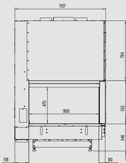
Vue du dessus
