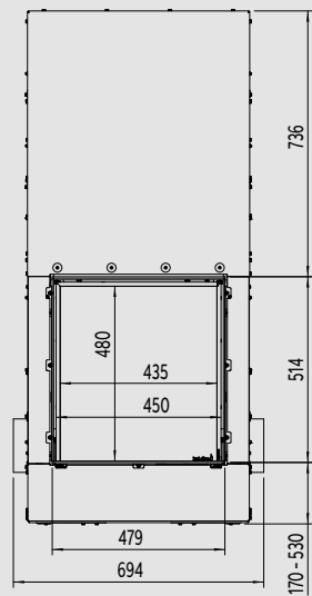
Vue du dessus
